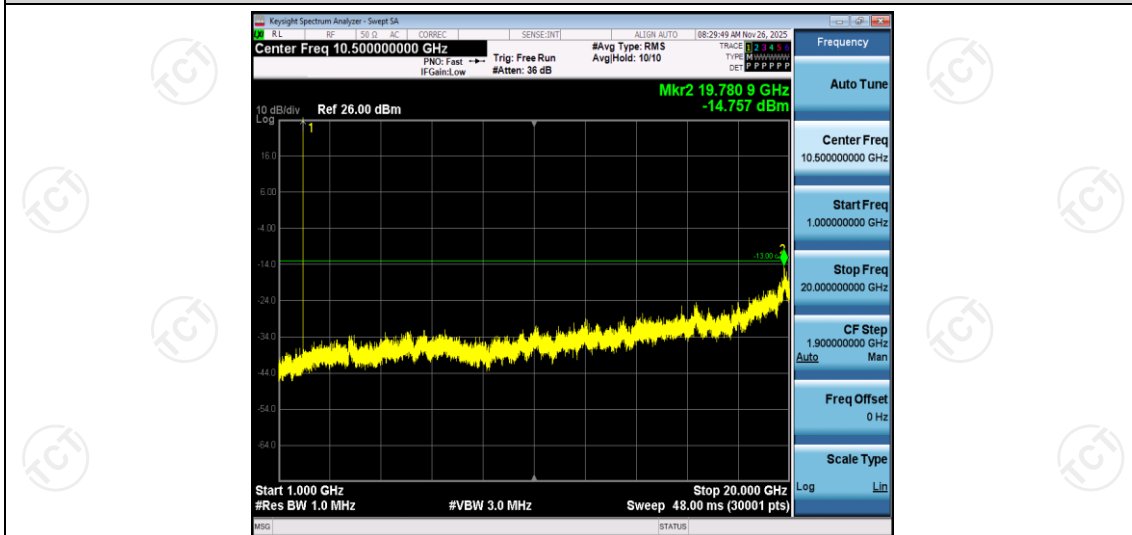
Band2-3MHz-QPSK-19185-1RB#0-Range2:1000~20000MHz
