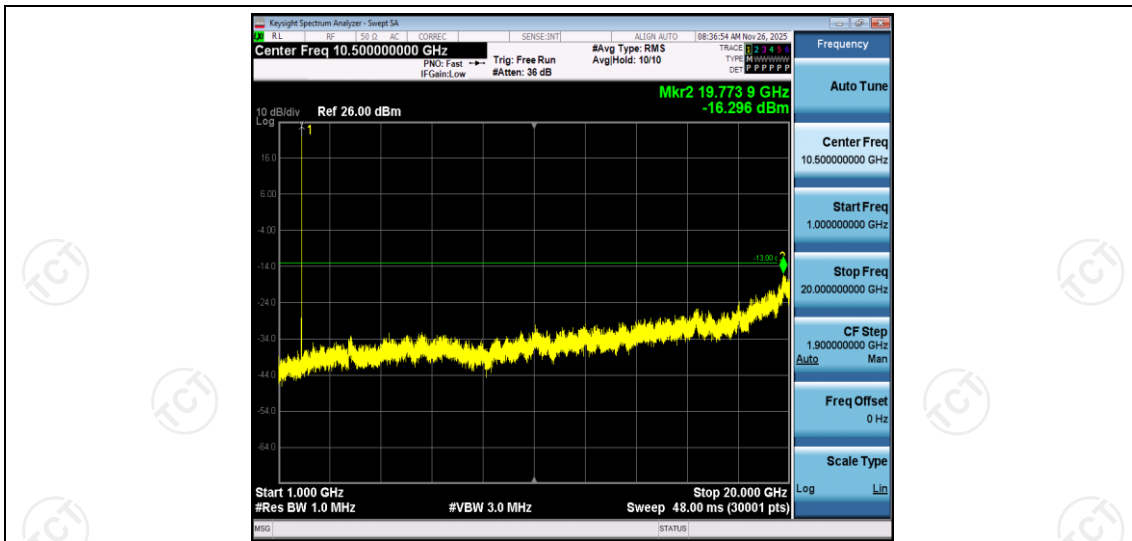
Band2-5MHz-QPSK-18625-1RB#0-Range2:1000~20000MHz
