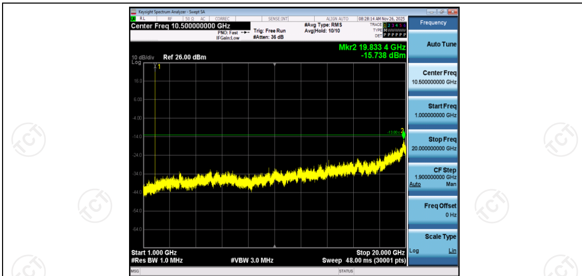
Band2-3MHz-16QAM-18615-1RB#0-Range2:1000~20000MHz
