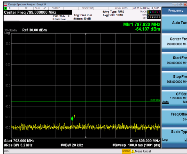
Band13-5MHz-QPSK-23255-1RB#0-Range4:793~805MHz
