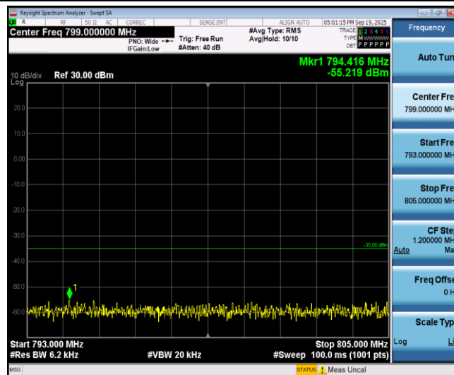
Band13-5MHz-QPSK-23230-1RB#0-Range4:793~805MHz
