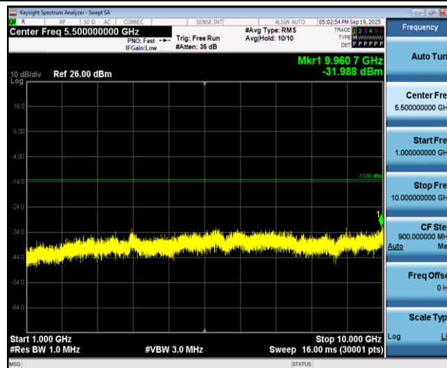
Band13-5MHz-QPSK-23255-1RB#0-Range2:1000~10000MHz
