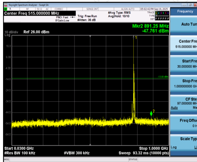
Band13-5MHz-QPSK-23255-1RB#0-Range1:30~1000MHz
