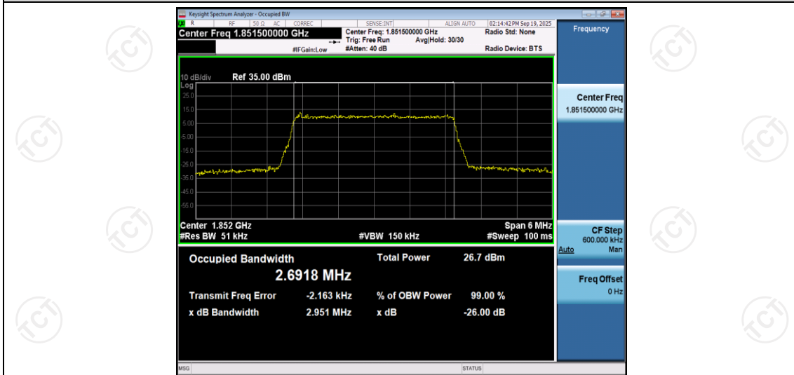
Band2-3MHz-QPSK-18615-15RB#0
