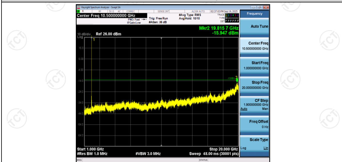
Band2-10MHz-QPSK-19150-1RB#0-Range2:1000~20000MHz
