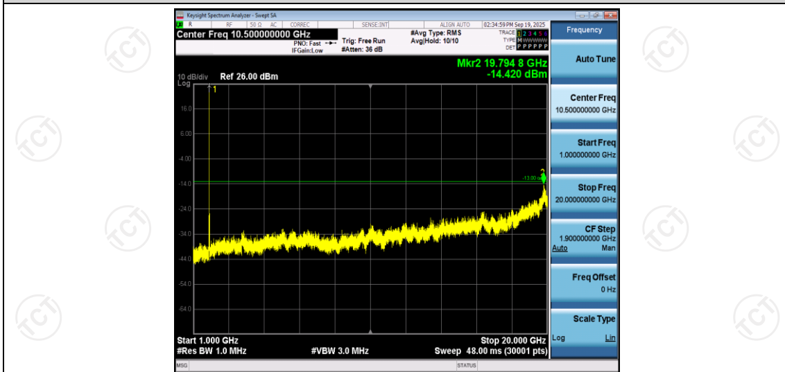
Band2-10MHz-QPSK-18650-1RB#0-Range2:1000~20000MHz
