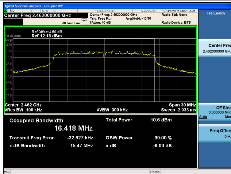
802.11n(HT20)_DTS_2412
