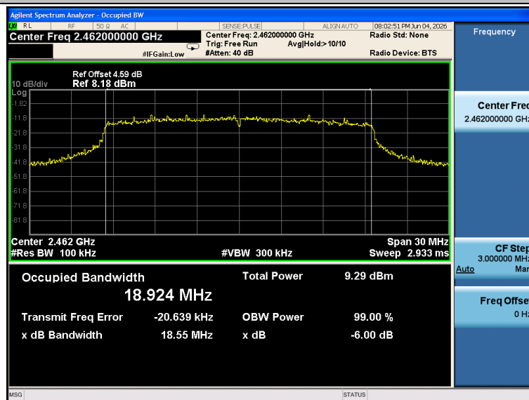
802.11n(HT40)_DTS_2422
