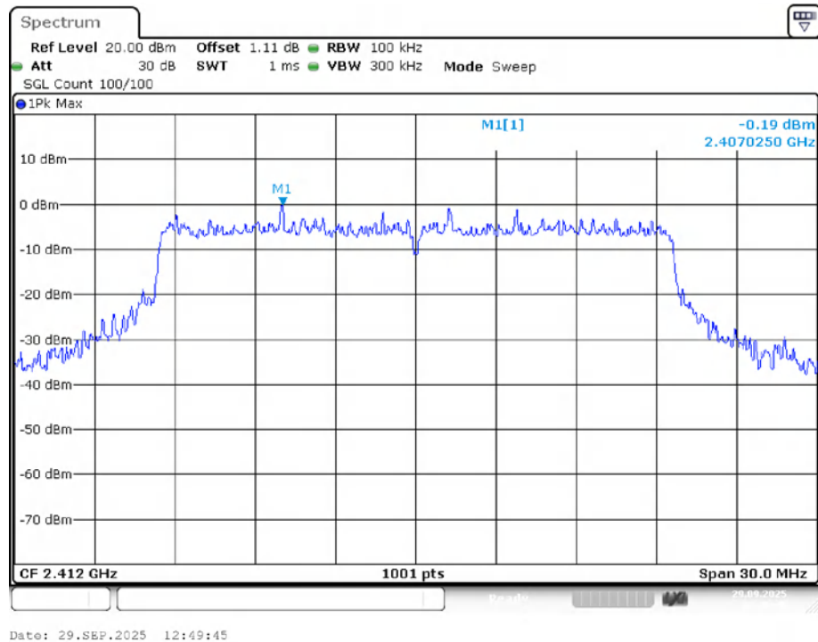
Band Edge NVNT ax20 2412MHz Ant1 Ref
