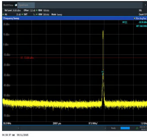
Band12-3MHz-QPSK-23025-15RB#0-30~1000-P ASS
