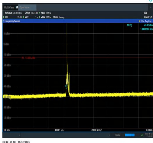
Band2-20MHz-16QAM-18700-1RB#0-1000~300 0-PASS
