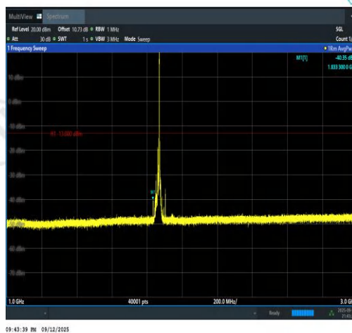
Band2-20MHz-16QAM-18700-1RB#99-1000~30
