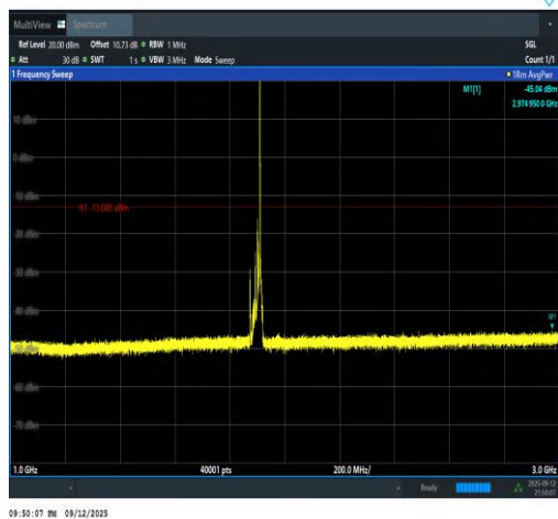
Band2-20MHz-QPSK-19100-1RB#99-1000~300 0-PASS
