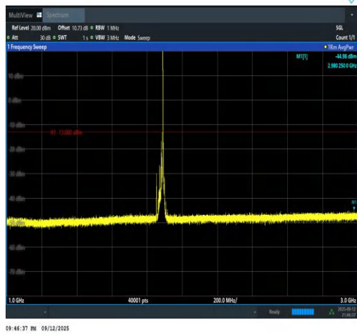
Band2-20MHz-QPSK-18900-1RB#99-1000~300
