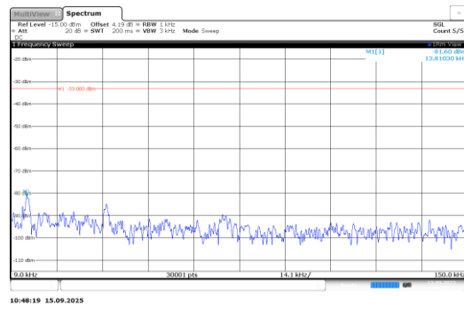
Band71-0.18-BPSK-133297-1@11-15kHz-0.009- 0.15-PASS
