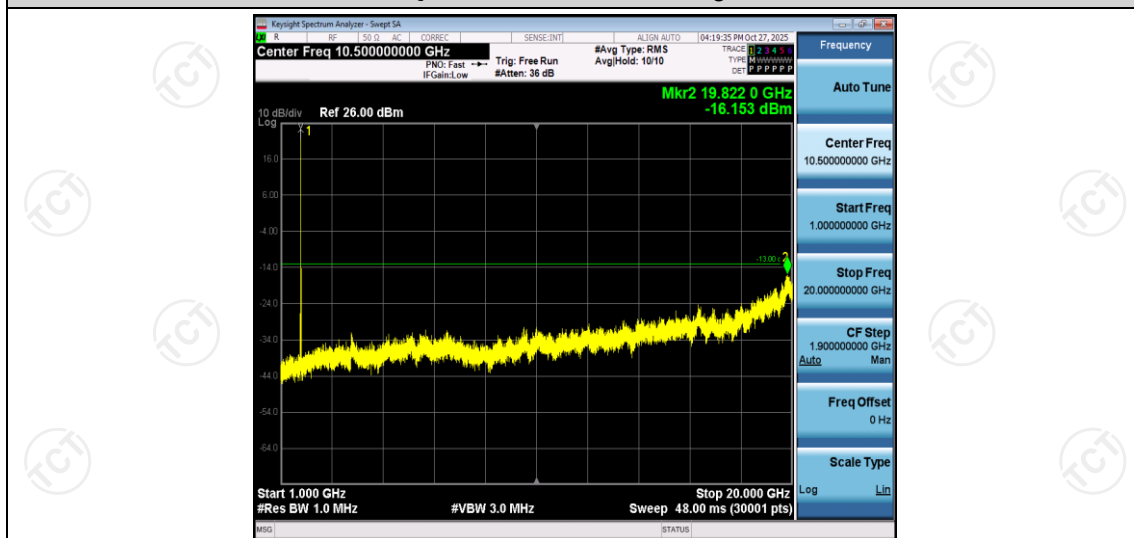
Band4-10MHz-QPSK-20350-1RB#0-Range2:1000~20000MHz
