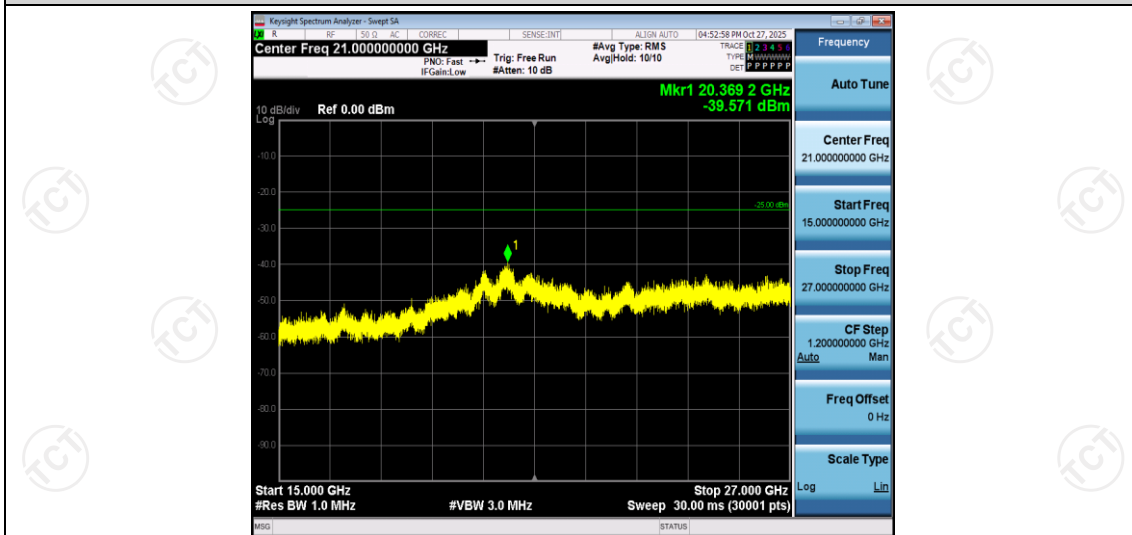
Band7-10MHz-QPSK-20800-1RB#0-Range3:15000~27000MHz
