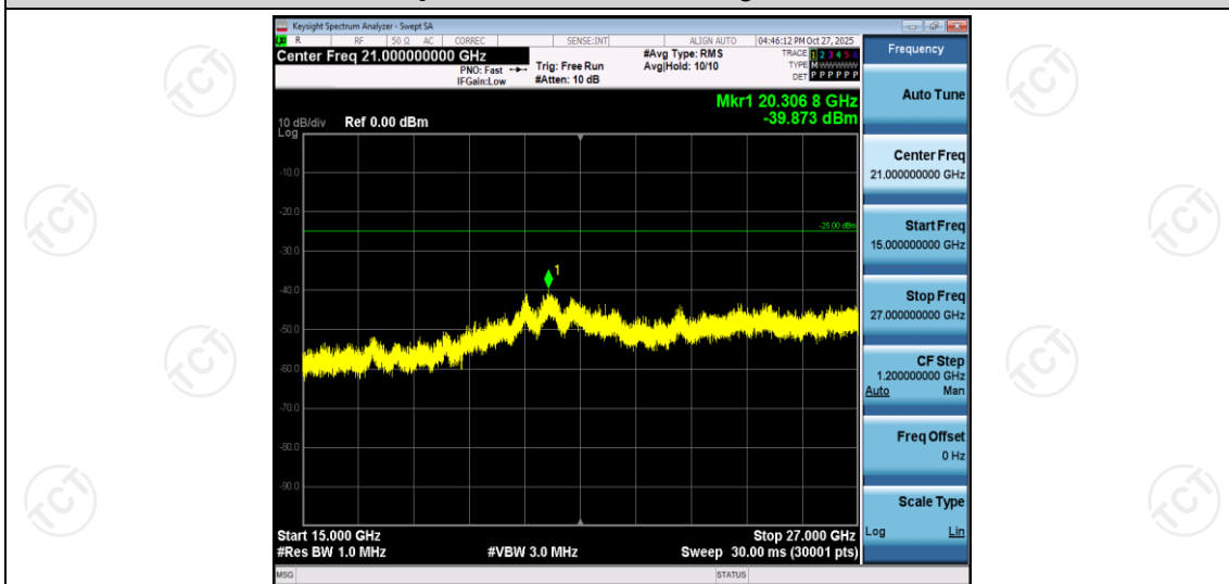
Band7-5MHz-QPSK-21425-1RB#0-Range3:15000~27000MHz
