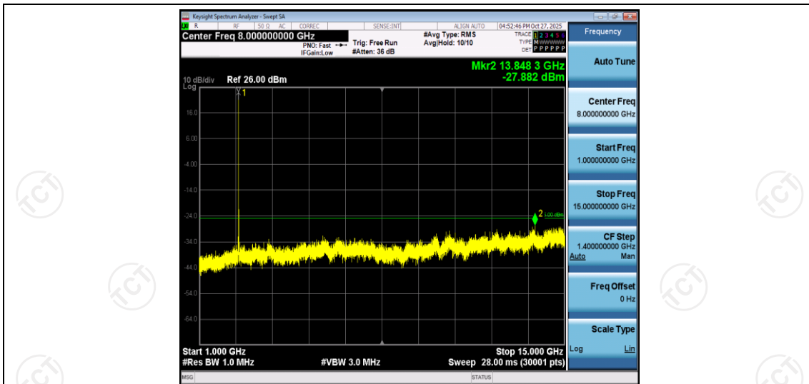
Band7-10MHz-QPSK-20800-1RB#0-Range2:1000~15000MHz
