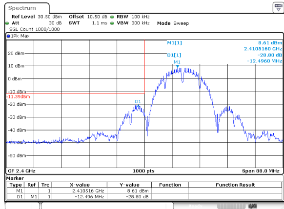
802.11b_2412MHz
