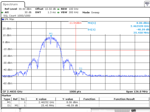
802.11b_2462MHz
