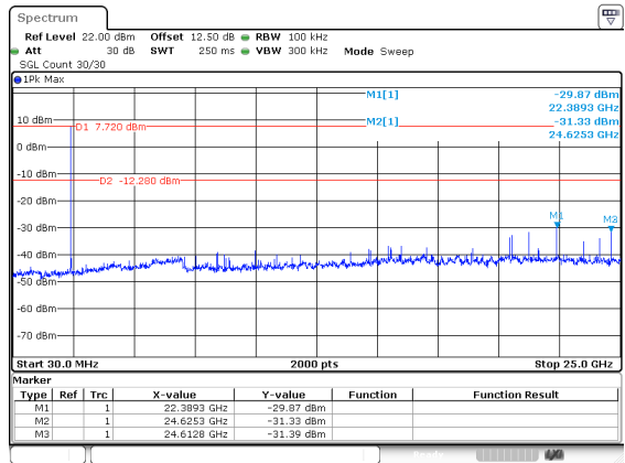
802.11b_2412MHz
