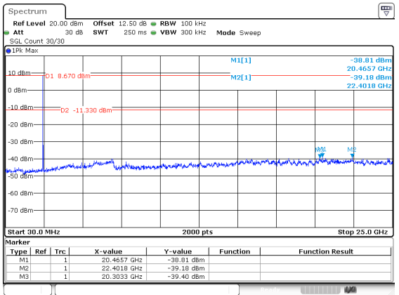
802.11b_2442MHz
