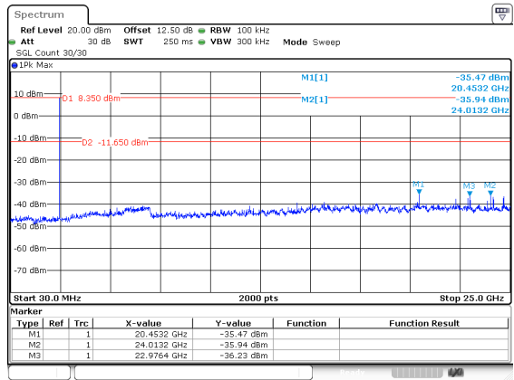
802.11b_2472MHz
