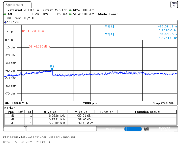
802.11b_2472MHz
