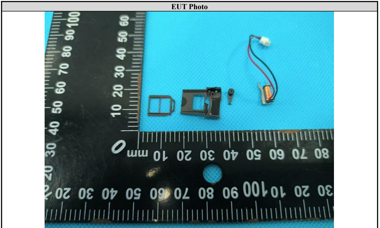
EUT Photo
