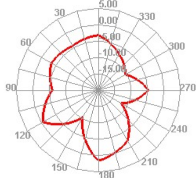
2400.000MHz E1
