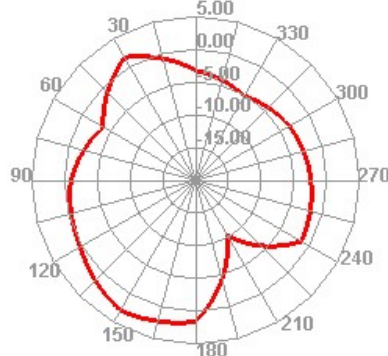
2400.000MHz E2
