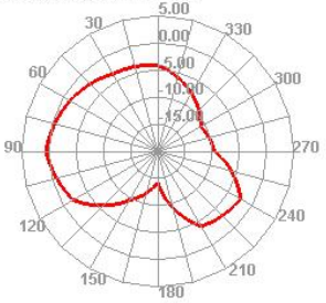
5550.000MHz E2
