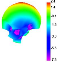
5350.000MHz E1
