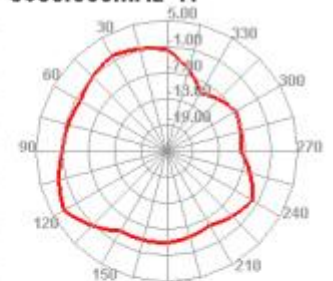
5650.000MHz H
