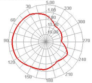
5450.000MHz H
