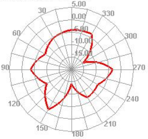
5550.000MHz E1
