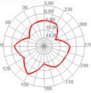
5650.000MHz E1
