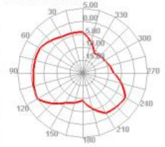
5650.000MHz E2
