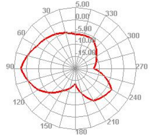
5450.000MHz E2
