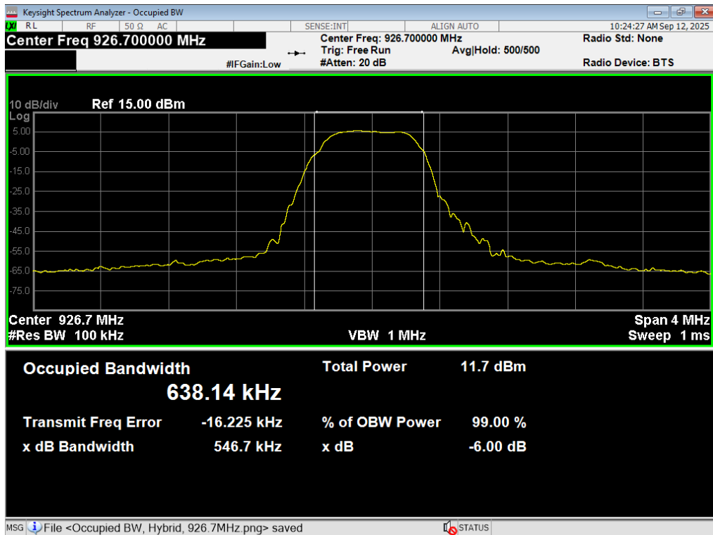
6dB BW, DTS, 926.7MHz
