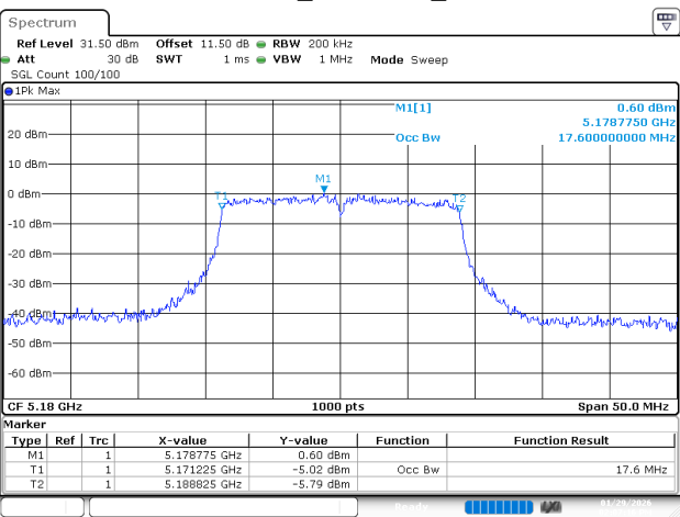
802.11ac20_5180MHz_Ant 2
