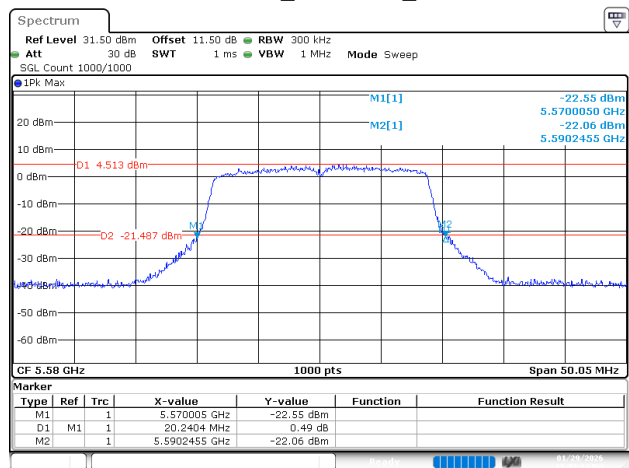
802.11ac20_5580MHz_Ant 1
