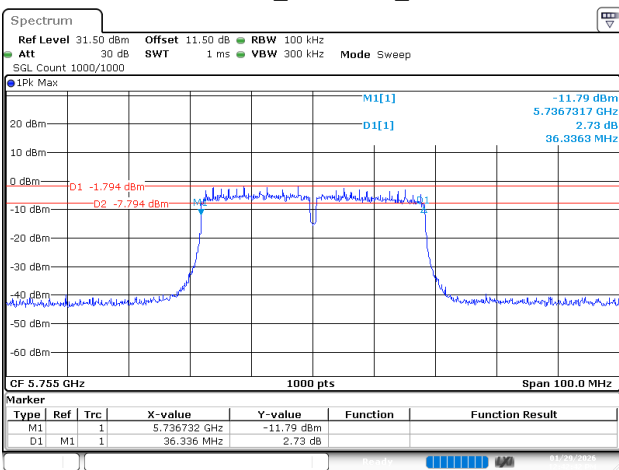
802.11ac40_5755MHz_Ant 1
