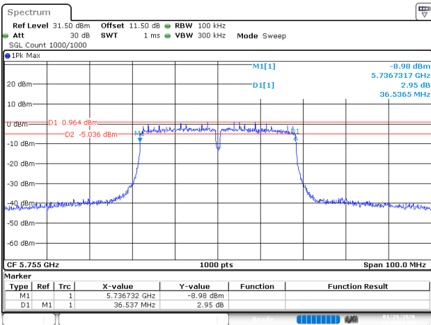
802.11ac40_5755MHz_Ant 2
