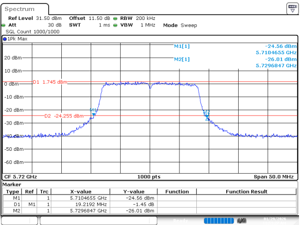
802.11a_5720MHz_Ant 1
