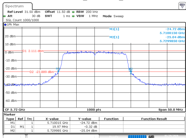
802.11ac20_5720MHz_Ant 1
