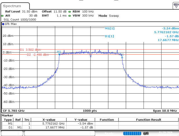
802.11ac20_5785MHz_Ant 2
