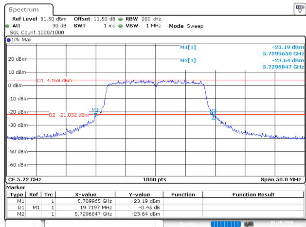
802.11a_5720MHz_Ant 2
