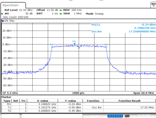
802.11ac20_5200MHz_Ant 2
