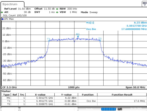
802.11ac20_5500MHz_Ant 2
