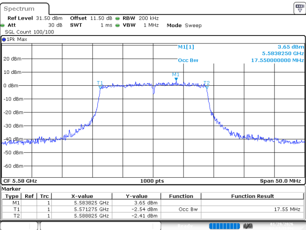
802.11ac20_5580MHz_Ant 2
