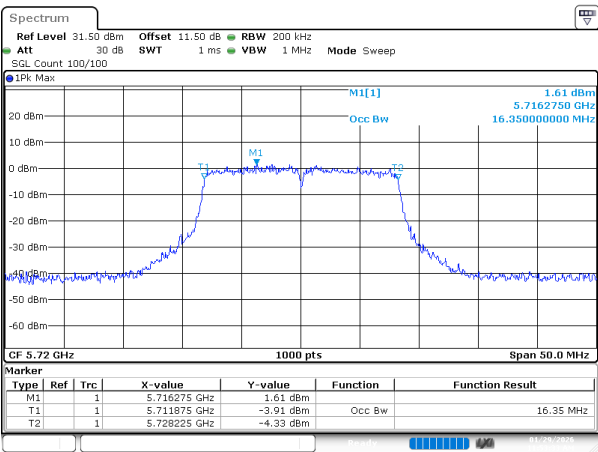
802.11a_5720MHz_Ant 1
