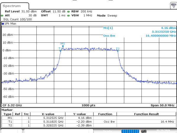
802.11a_5320MHz_Ant 2
