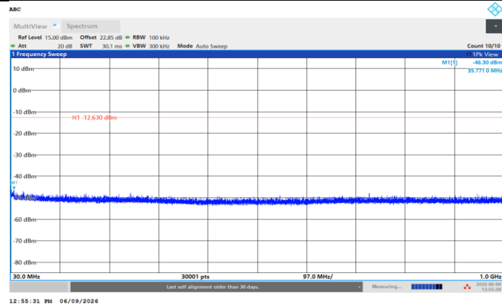
BLE_2M_Ant2_2480_30~1000
