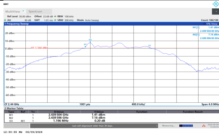
BLE_2M_Ant2_2440
