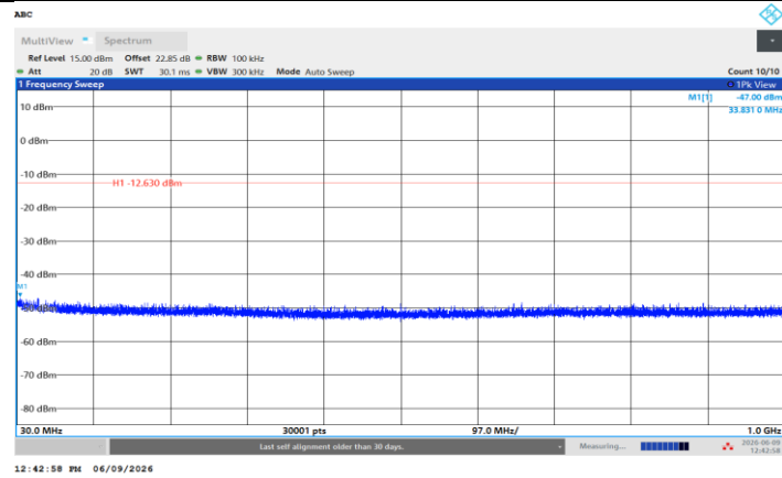
BLE_1M_Ant2_2480_30~1000
