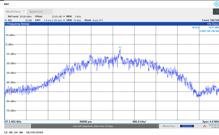
BLE_2M_Ant2_2402
