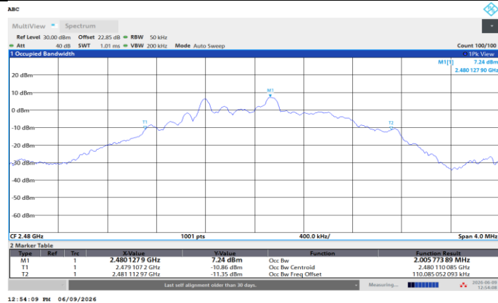
BLE_2M_Ant2_2480
