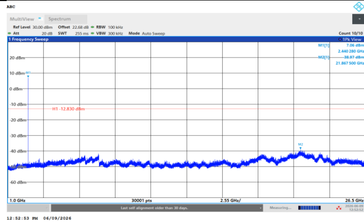
BLE_2M_Ant2_2440_1000~26500
