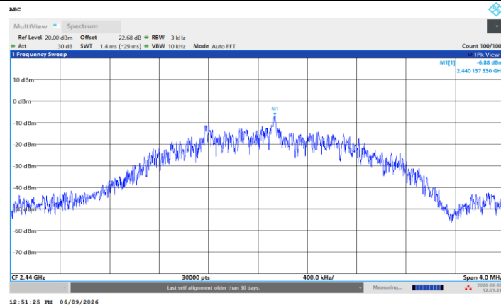
BLE_2M_Ant2_2440
