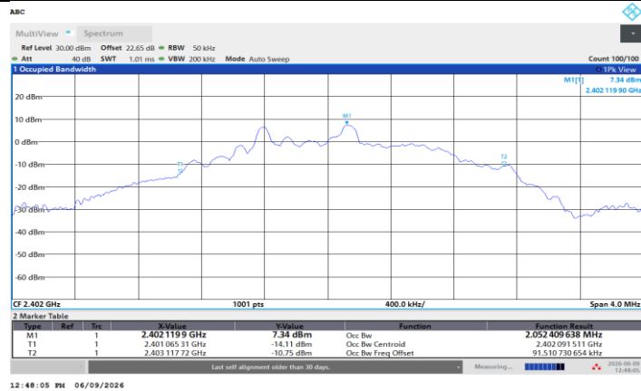
BLE_2M_Ant2_2402
