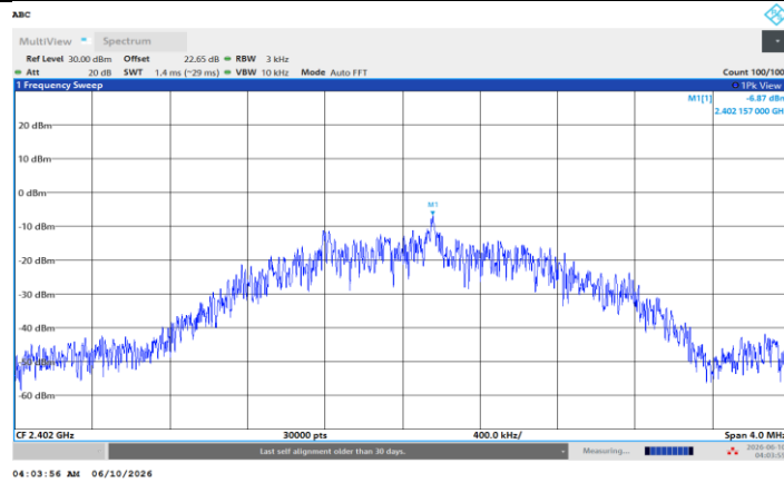
BLE_2M_Ant1_2402
