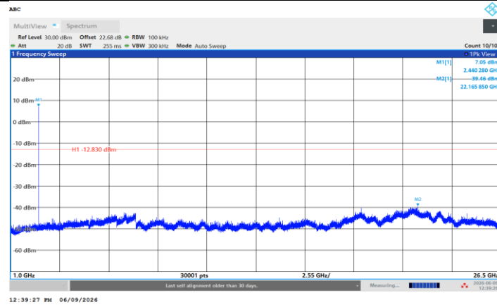
BLE_1M_Ant2_2440_1000~26500
