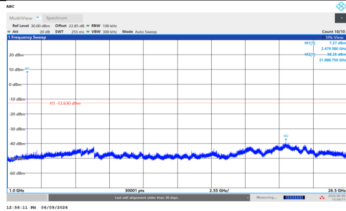
BLE_2M_Ant2_2480_1000~26500
