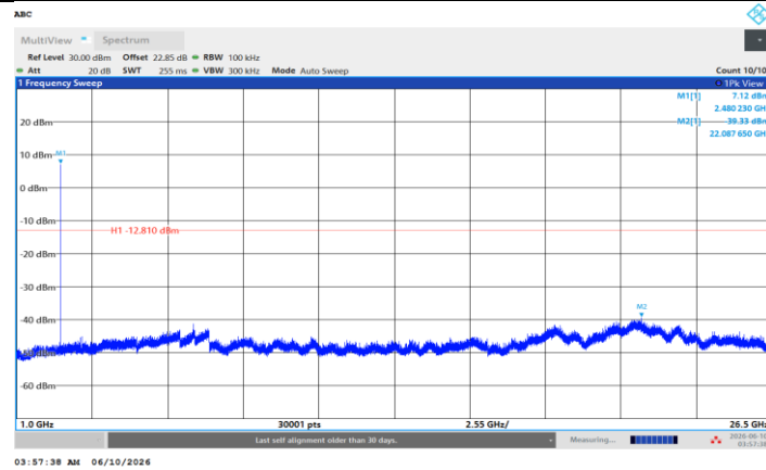
BLE_1M_Ant1_2480_1000~26500
