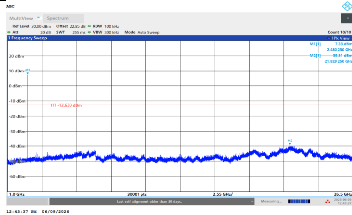
BLE_1M_Ant2_2480_1000~26500
