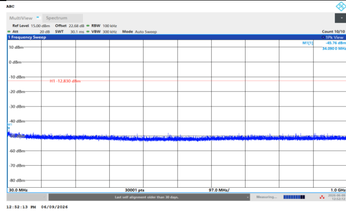
BLE_2M_Ant2_2440_30~1000
