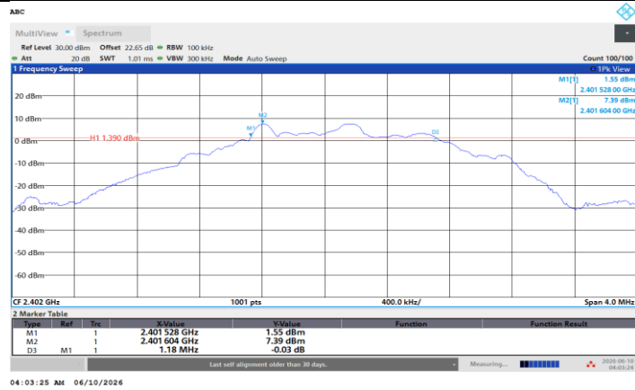
BLE_2M_Ant1_2402
