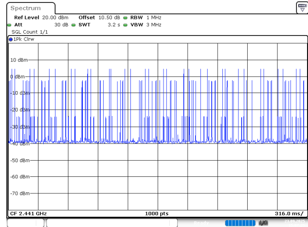
3EDR_DH1_Hopping
