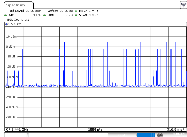
3EDR_DH5_Hopping
