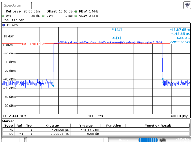
3EDR_DH5_Hopping
