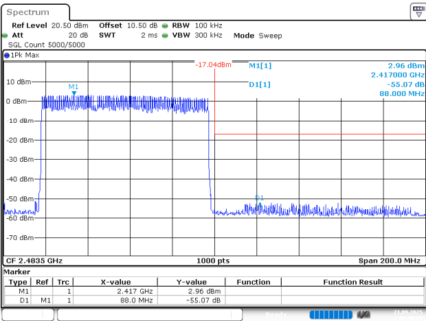
3EDR_DH1_Hopping_Upper
