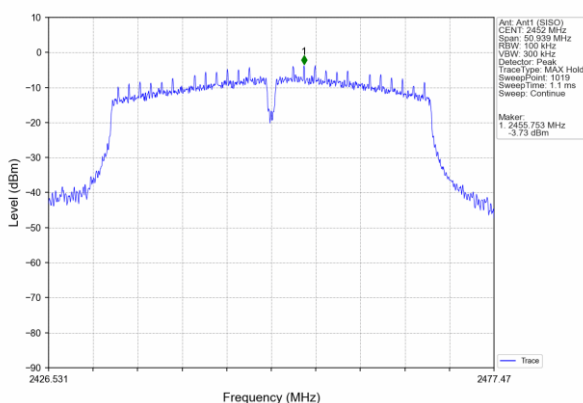
802.11n40 2452MHz
