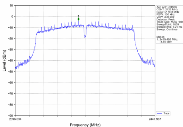
802.11n 40 2422MHz
