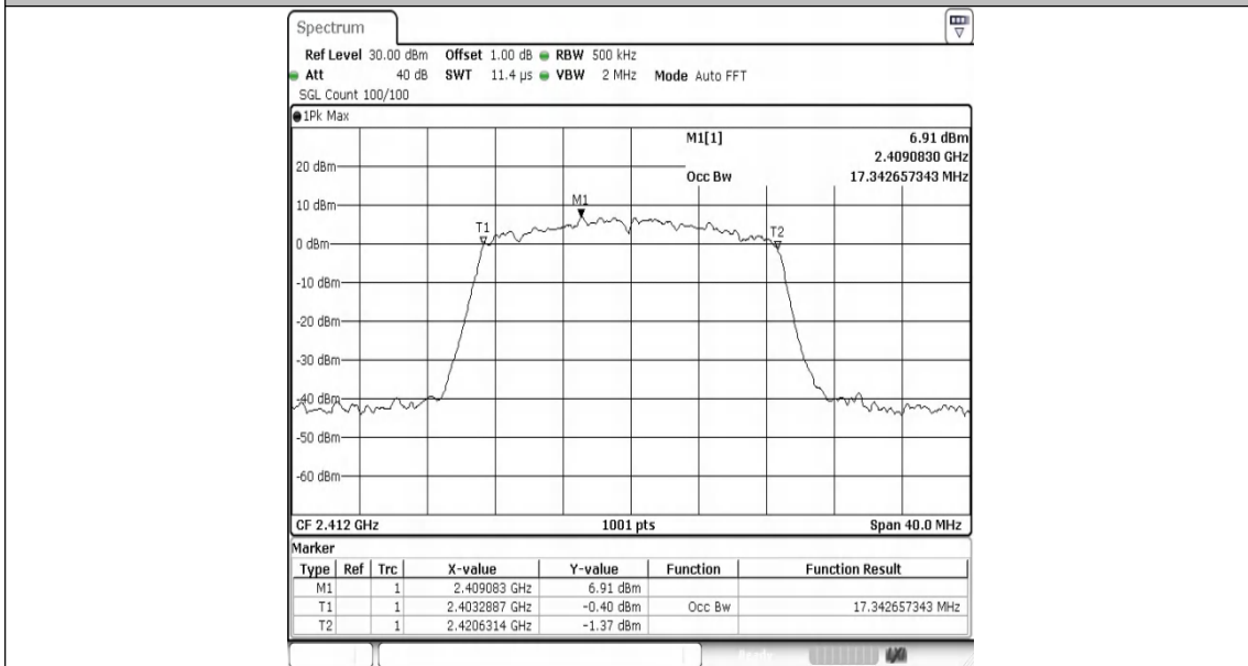
11N20MIMO-Ant0-2412
