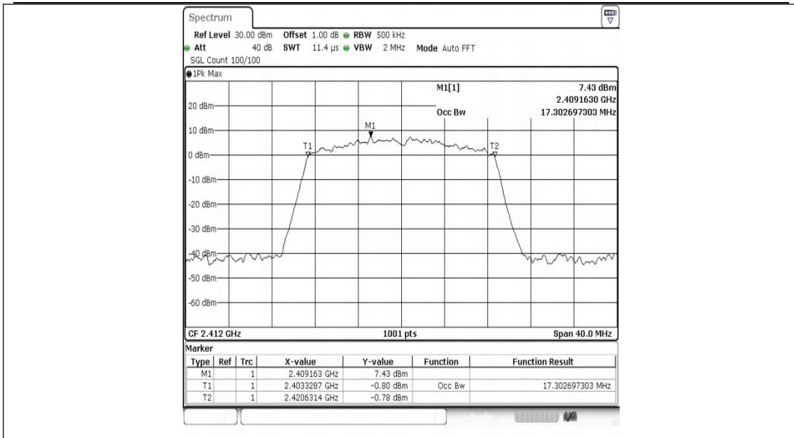
11N20MIMO-Ant0-2412
