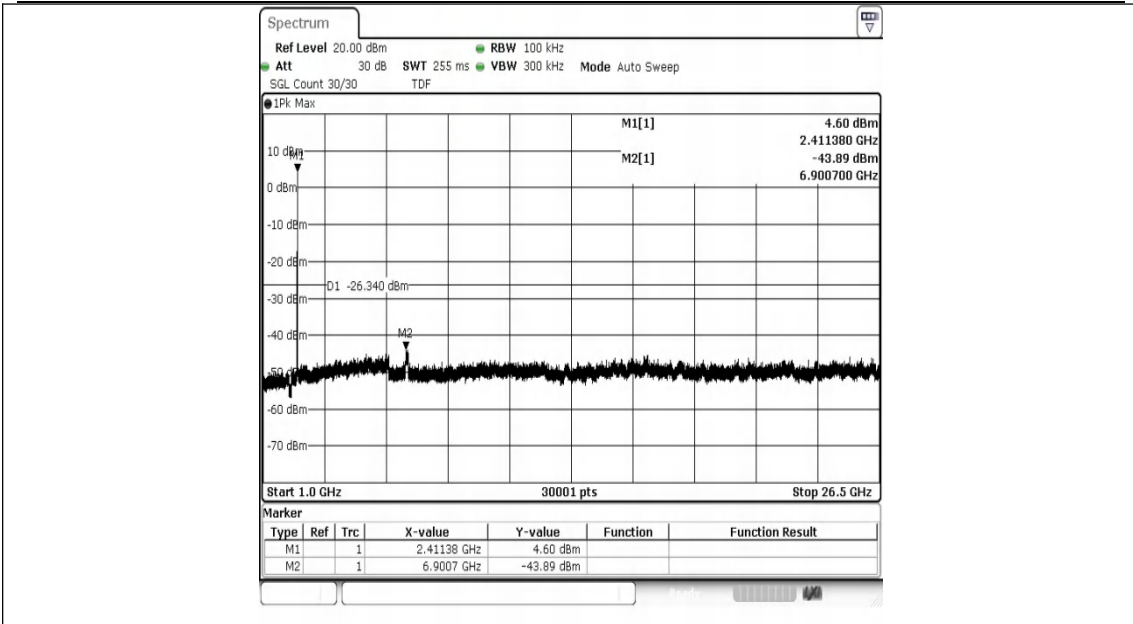
11B-Ant0-2412-1000~26500-PASS
