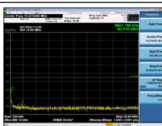
Band41(2535-2655)-5MHz-QPSK-40640-1RB#0- 0.15~30-PASS
