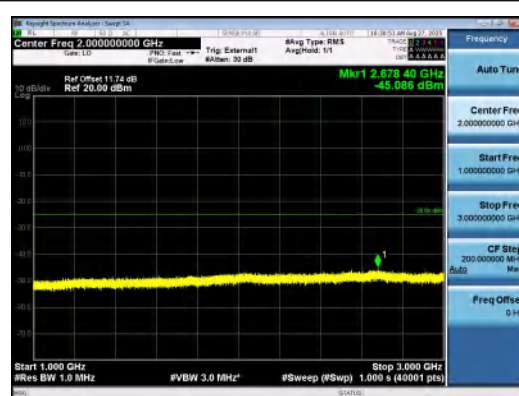
Band41(2535-2655)-10MHz-16QAM-40090-1RB #49-1000~3000-PASS
