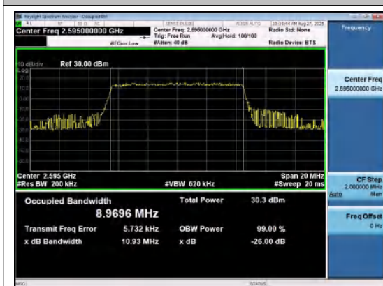
Band41(2535-2655)-10MHz-QPSK-40640-50RB# 0-PASS
