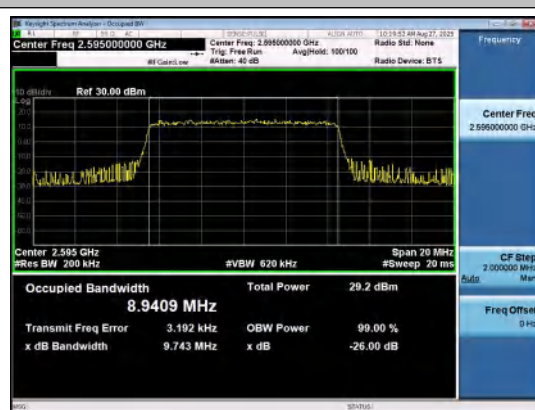
Band41(2535-2655)-10MHz-16QAM-40640-50RB# 0-PASS
