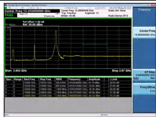
Band41(2535-2655)-10MHz-QPSK-41190-1RB#49 -PASS
