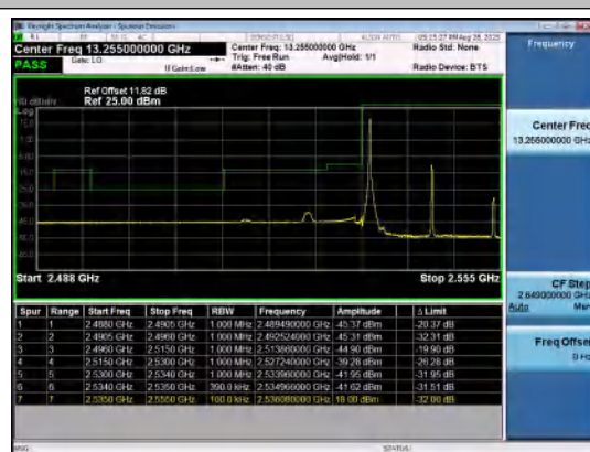
Band41(2535-2655)-20MHz-16QAM-40140-1RB#0 -PASS
