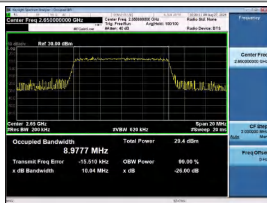
Band41(2535-2655)-10MHz-16QAM-41190-50RB# 0-PASS
