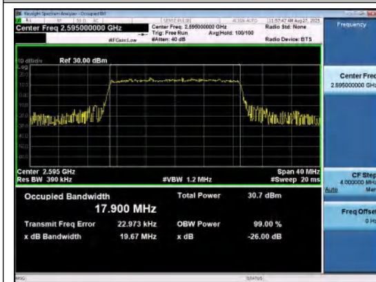
Band41(2535-2655)-20MHz-QPSK-40640-100RB #0-PASS
