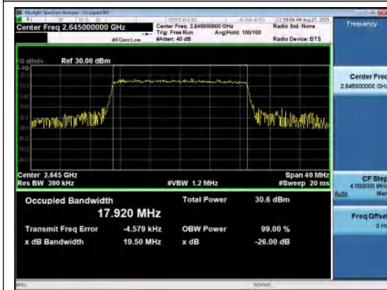
Band41(2535-2655)-20MHz-QPSK-41140-100RB #0-PASS
