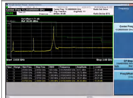
Band41(2535-2655)-20MHz-16QAM-41140-1RB#99 99-PASS
