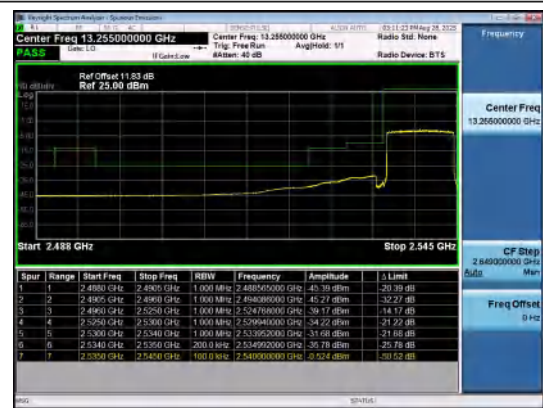
Band41(2535-2655)-10MHz-16QAM-40090-50RB# 0-PASS
