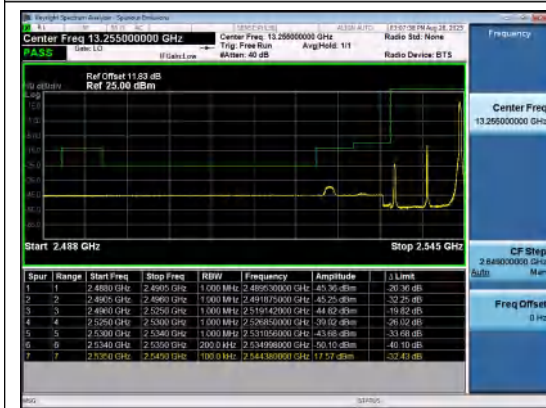
Band41(2535-2655)-10MHz-16QAM-40090-1RB# 49-PASS
