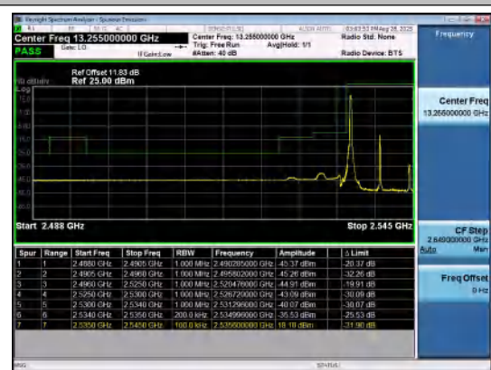
Band41(2535-2655)-10MHz-16QAM-40090-1RB#0 -PASS
