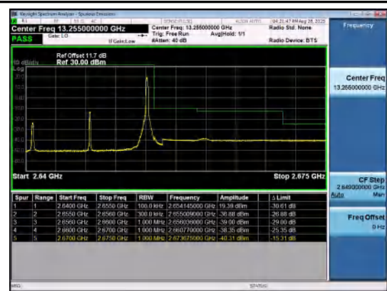
Band41(2535-2655)-15MHz-QPSK-41165-1RB#74 -PASS
