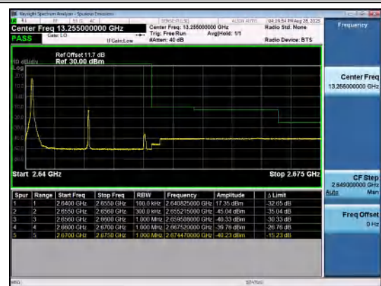
Band41(2535-2655)-15MHz-16QAM-41165-1RB#0 -PASS
