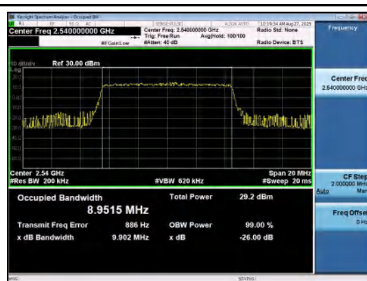
Band41(2535-2655)-10MHz-16QAM-40090-50RB# 0-PASS
