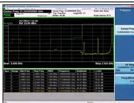
Band41(2535-2655)-20MHz-QPSK-40140-1RB#99 -PASS
