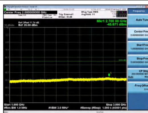
Band41(2535-2655)-5MHz-QPSK-40640-1RB#0- 1000~3000-PASS
