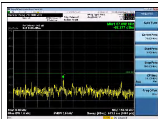
Band41(2535-2655)-5MHz-QPSK-40640-1RB#0- 0.009~0.15-PASS
