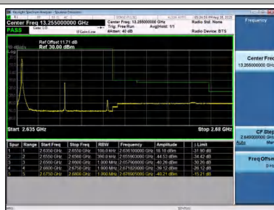
Band41(2535-2655)-20MHz-16QAM-41140-1RB#0 -PASS
