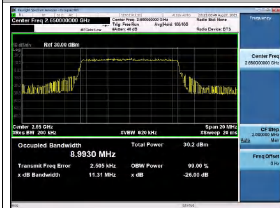
Band41(2535-2655)-10MHz-QPSK-41190-50RB# 0-PASS
