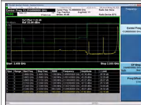
Band41(2535-2655)-20MHz-16QAM-40140-1RB#99 99-PASS
