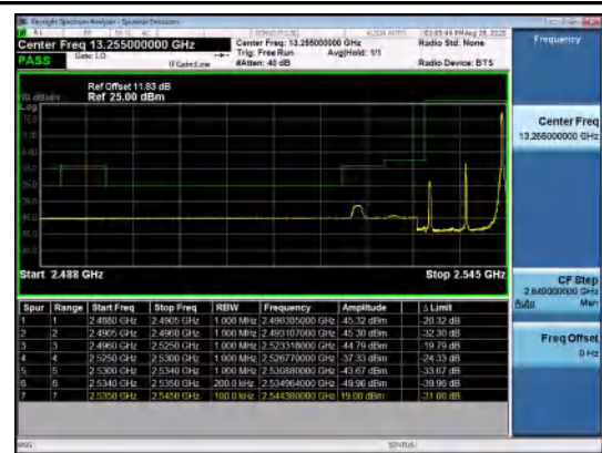
Band41(2535-2655)-10MHz-QPSK-40090-1RB#49 -PASS
