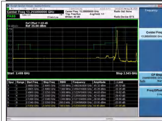
Band41(2535-2655)-10MHz-QPSK-40090-1RB#0 -PASS
