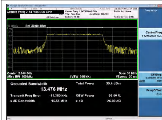
Band41(2535-2655)-15MHz-QPSK-41165-75RB# 0-PASS
