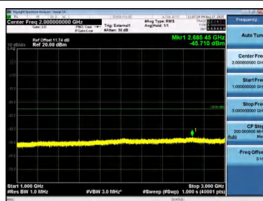
Band41(2535-2655)-20MHz-16QAM-40140-1RB #99-1000~3000-PASS
