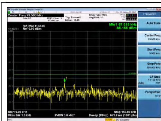
Band41(2535-2655)-20MHz-16QAM-40640-1RB #99-0.009~0.15-PASS
