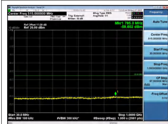
Band41(2535-2655)-20MHz-16QAM-40640-1RB #99-30~1000-PASS
