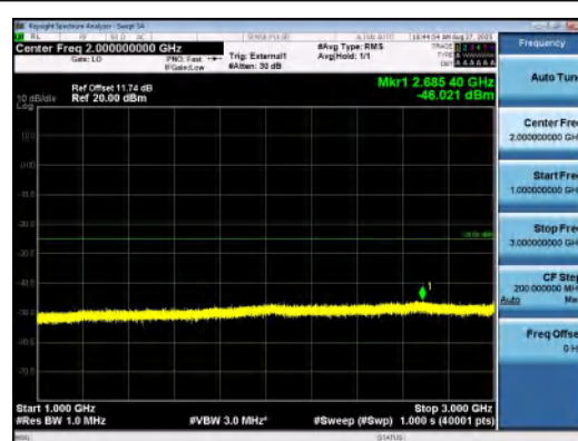
Band41(2535-2655)-10MHz-QPSK-40640-1RB# 49-1000~3000-PASS
