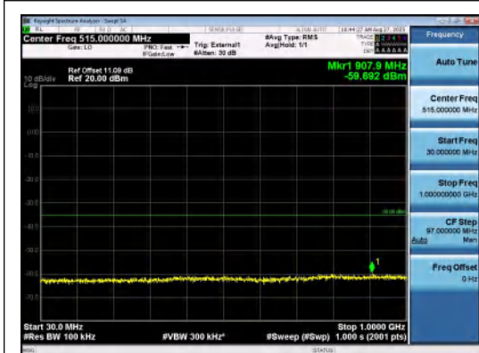
Band41(2535-2655)-10MHz-QPSK-40640-1RB# 49-30~1000-PASS
