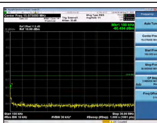
Band41(2535-2655)-10MHz-QPSK-40640-1RB# 49-0.15~30-PASS
