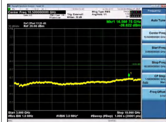
Band41(2535-2655)-20MHz-16QAM-40640-1RB #99-3000~18000-PASS
