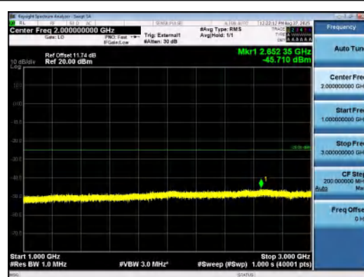
Band41(2535-2655)-20MHz-16QAM-40640-1RB #99-1000~3000-PASS
