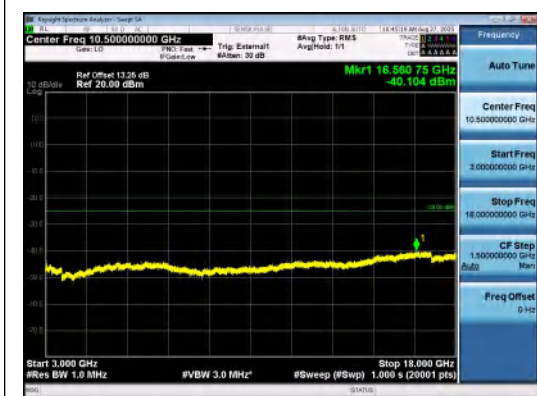
Band41(2535-2655)-10MHz-QPSK-40640-1RB# 49-3000~18000-PASS
