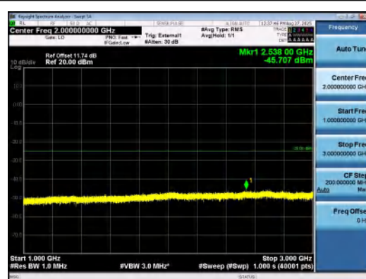
Band41(2535-2655)-20MHz-16QAM-41140-1RB #99-1000~3000-PASS
