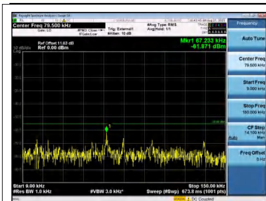
Band41(2535-2655)-10MHz-QPSK-40640-1RB# 49-0.009~0.15-PASS
