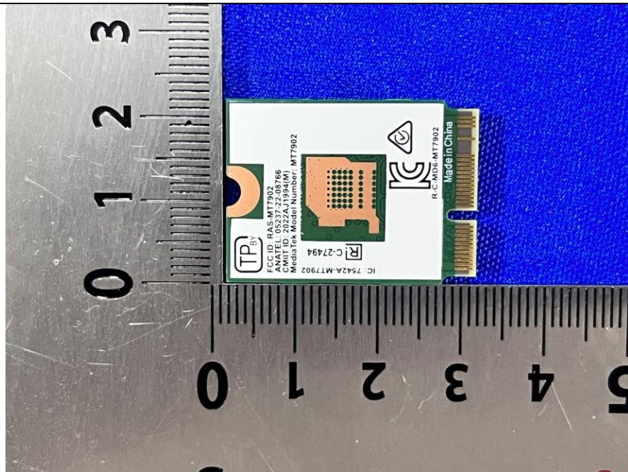
(FCC ID:RAS-MT7902)
