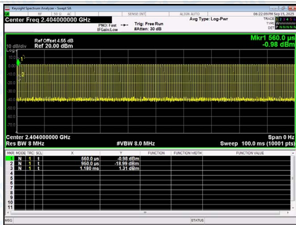
Duty Cycle NVNT BLE 2Mbps 2404MHz Ant1
