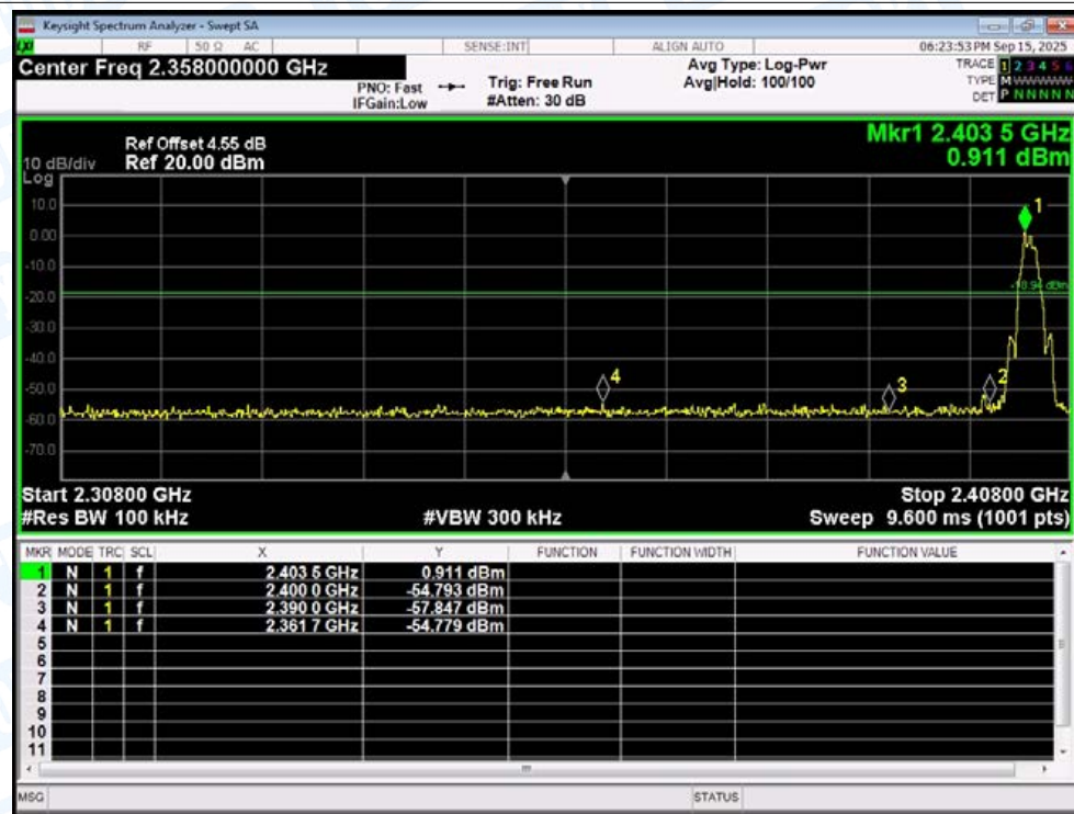
Band Edge NVNT BLE 2Mbps 2404MHz Ant1 Emission
