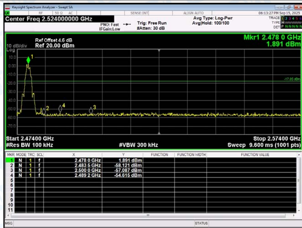
Band Edge NVNT BLE 2Mbps 2478MHz Ant1 Emission
