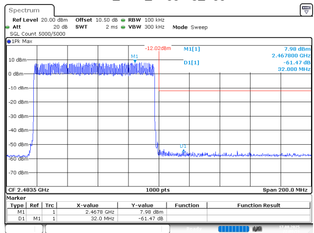
2EDR_DH1_Hopping_Upper
