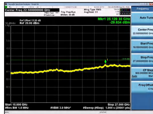
Band7-15MHz-16QAM-20825-1RB#74-18000~27000-P ASS
