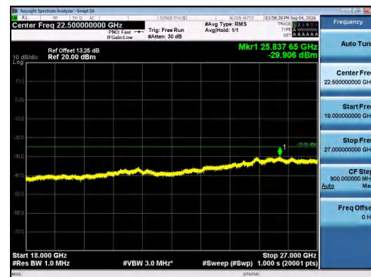
Band7-20MHz-QPSK-21350-1RB#0-18000~27000-PAS
