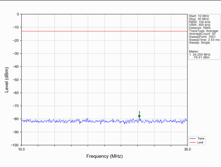
Band2_10MHz_16QAM_MCH_1880MHz_RB_1_0_NTNV
