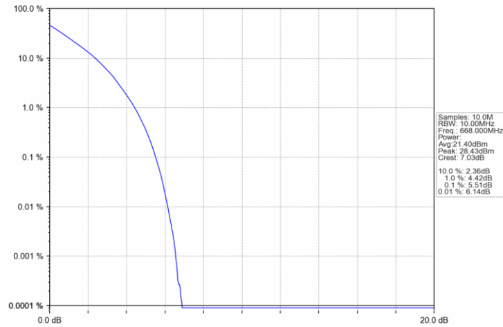
Band71 10MHz QPSK LCH 668MHz RB 50 0 NTN
