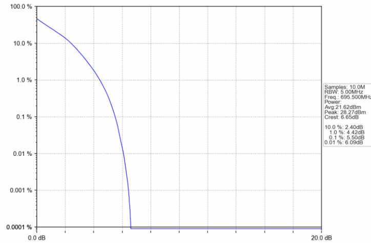
Band71 5MHz QPSK HCH 695.5MHz RB 25 0 NTNV
