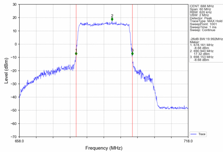
Band71 20MHz 16QAM HCH 688MHz RB 100 0 NTNV
