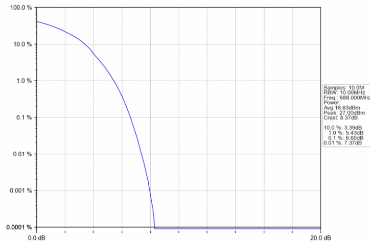
Band71 20MHz 16QAM HCH 688MHz RB 100 0 NTNV
