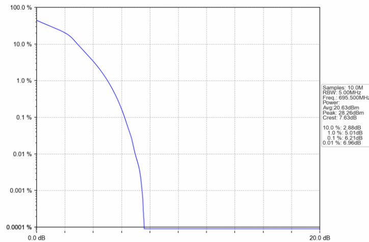
Band71 5MHz 16QAM HCH 695.5MHz RB 25 0 NTNV
