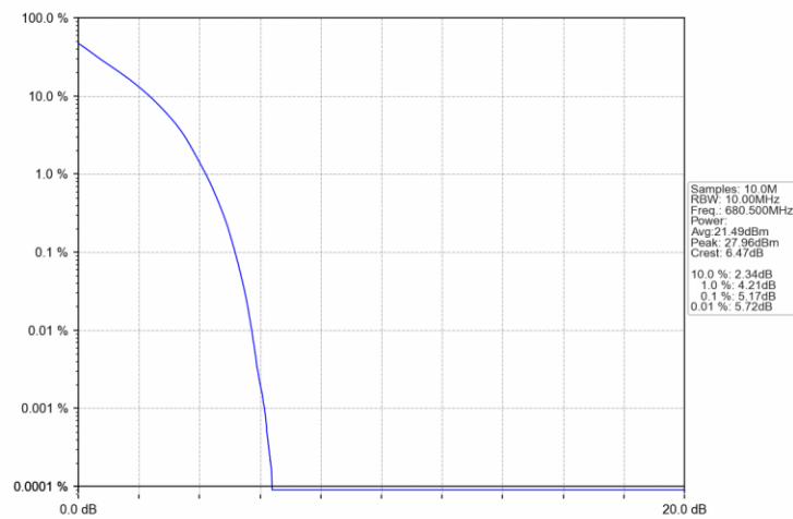
Band71 10MHz QPSK MCH 680.5MHz RB 50 0 NTN
