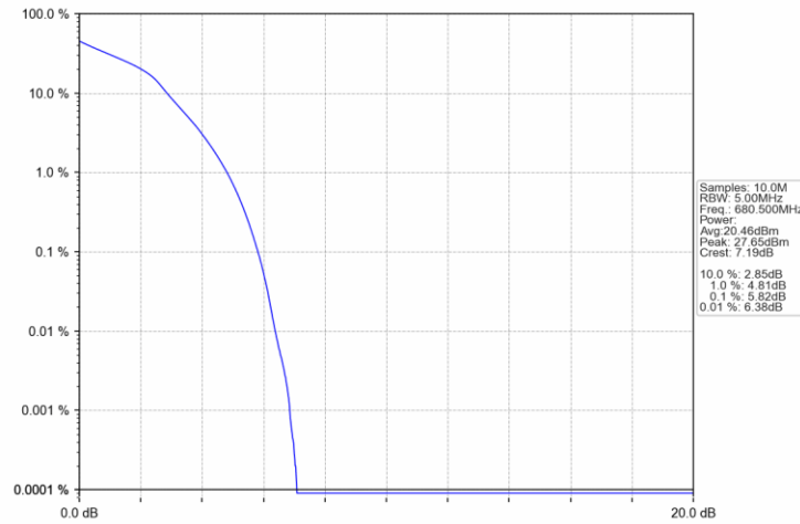
Band71 5MHz 16QAM MCH 680.5MHz RB 25 0 NTNV
