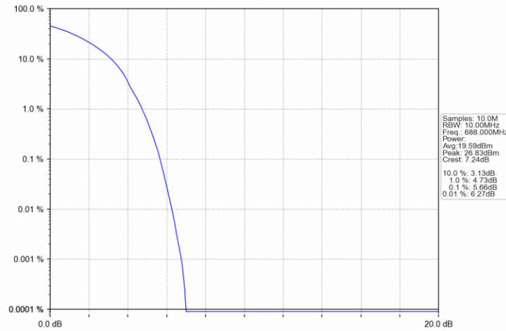
Band71 20MHz QPSK HCH 688MHz RB 100 0 NTNV
