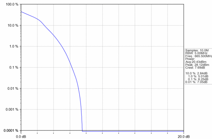
Band71 5MHz 16QAM LCH 665.5MHz RB 25 0 NTNV
