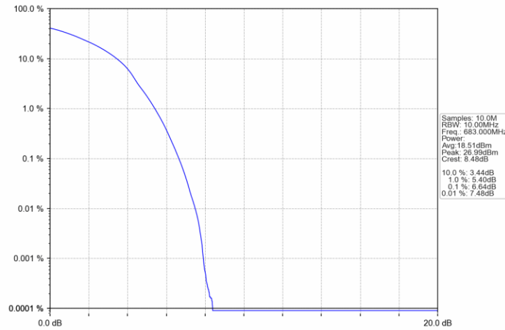
Band71 20MHz 16QAM MCH 683MHz RB 100 0 NTNV
