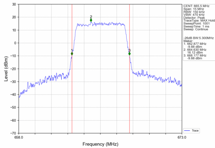
Band71 5MHz 16QAM LCH 665.5MHz RB 25 0 NTN
