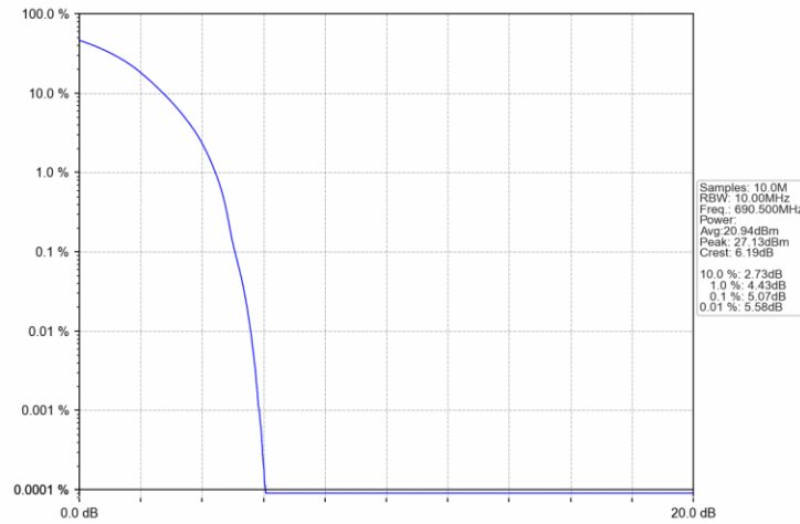
Band71 15MHz QPSK HCH 690.5MHz RB 75 0 NTNV
