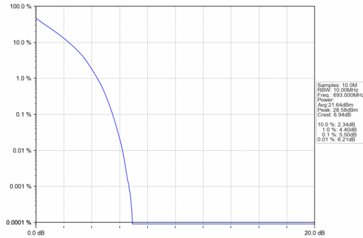
Band71 10MHz QPSK HCH 693MHz RB 50 0 NTN
