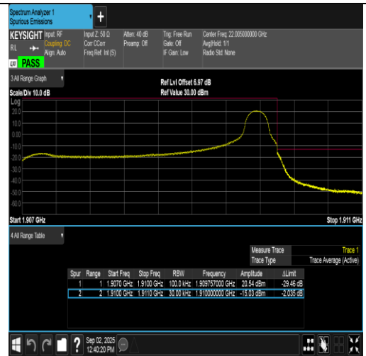
Band2-3MHz-QPSK-19185-1RB#14-PASS
