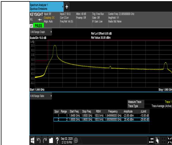
Band2-10MHz-QPSK-18650-1RB#0-PASS
