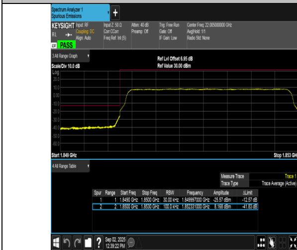
Band2-3MHz-QPSK-18615-15RB#0-PASS
