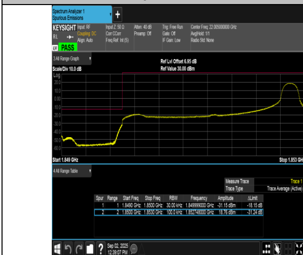
Band2-3MHz-16QAM-18615-1RB#14-PASS
