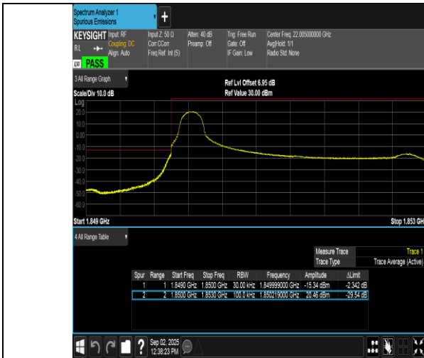
Band2-3MHz-QPSK-18615-1RB#0-PASS
