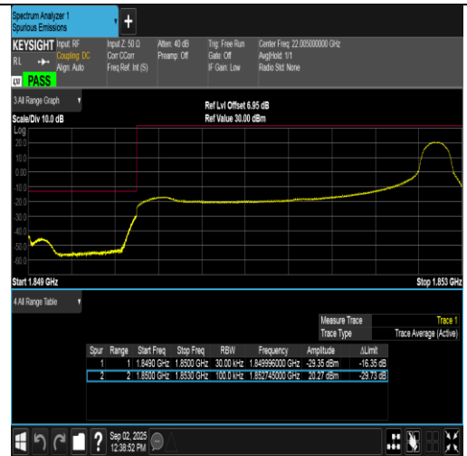
Band2-3MHz-QPSK-18615-1RB#14-PASS
