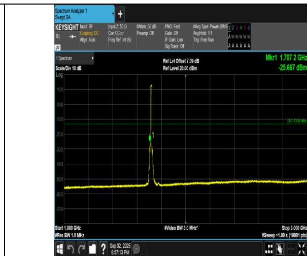
Band4-10MHz-QPSK-20000-50RB#0-1000~3000-PASS
