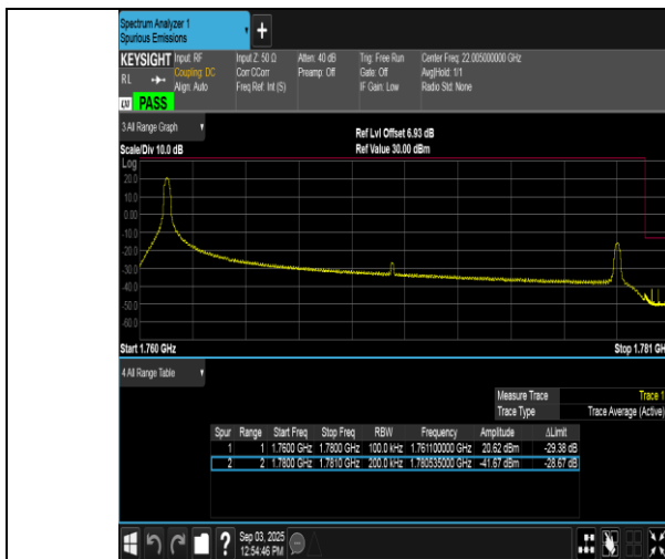
Band66-20MHz-QPSK-132572-1RB#0-PASS
