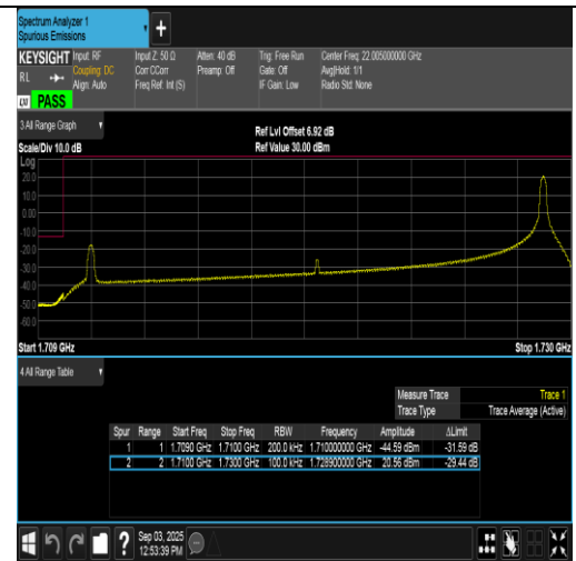
Band66-20MHz-QPSK-132072-1RB#99-PASS
