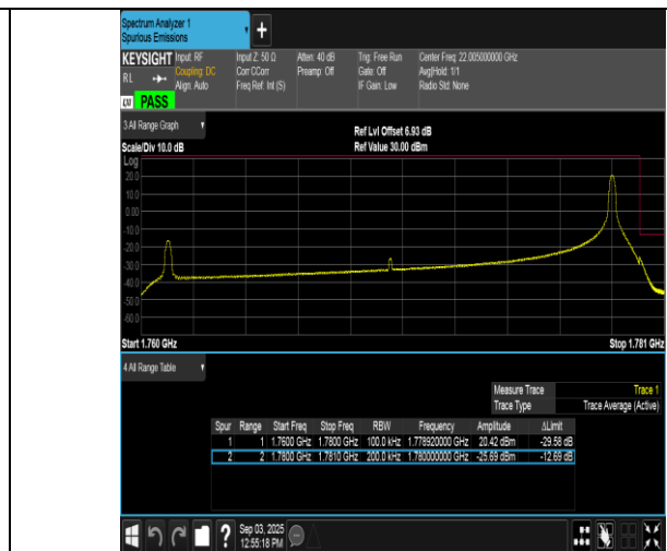
Band66-20MHz-QPSK-132572-1RB#99-PASS
