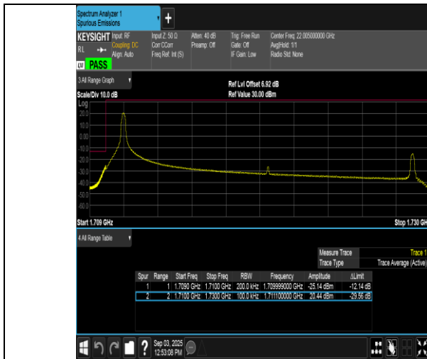
Band66-20MHz-QPSK-132072-1RB#0-PASS
