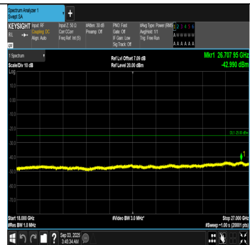
Band7-20MHz-QPSK-21100-1RB#99-18000~27000-PASS
