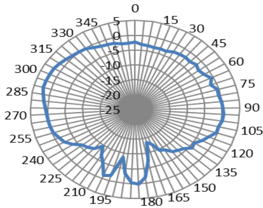
XZ-5500MHz
