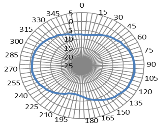
XY-2450MHz
