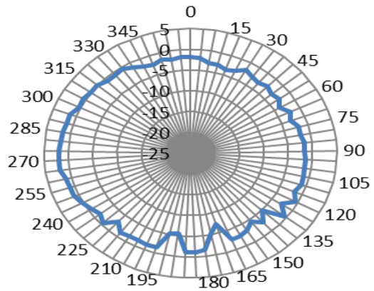
YZ-5500MHz
