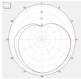
BLUETOOTH_Tis_Rssi_H39 Polar
