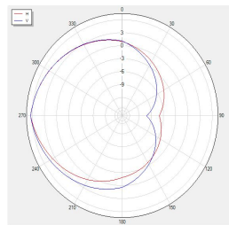
BLUETOOTH_Trp_V39 Polar
