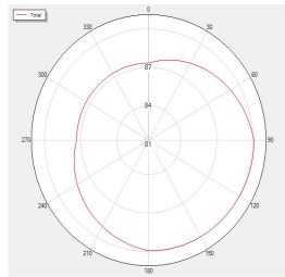
BLUETOOTH_Tis_Rssi_H78 Total
