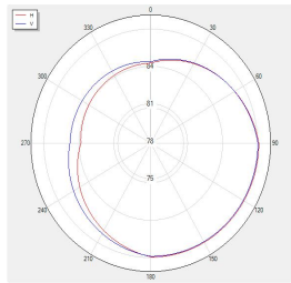
BLUETOOTH_Tis_Rssi_H78 Polar
