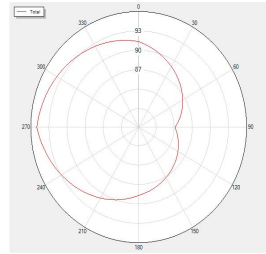
BLUETOOTH_Tis_Rssi_V78 Total
