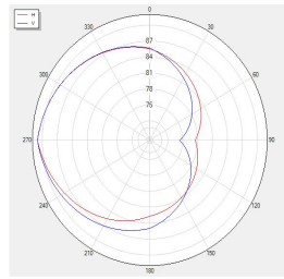
BLUETOOTH_Tis_Rssi_V39 Polar
