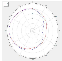
BLUETOOTH_Tis_Rssi_V78 Polar
