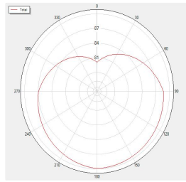
BLUETOOTH_Tis_Rssi_H39 Total
