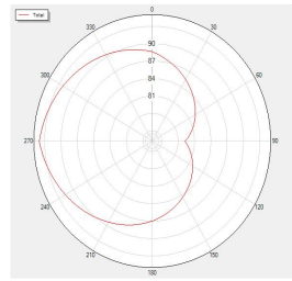
BLUETOOTH_Tis_Rssi_V39 Total
