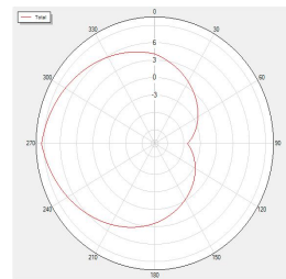
BLUETOOTH_Trp_V39 Total
