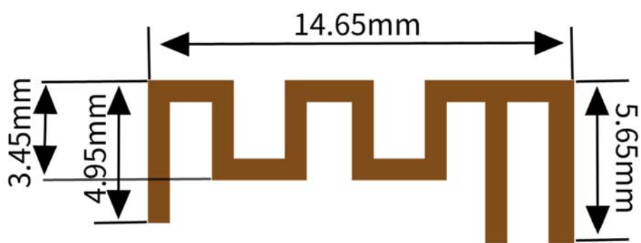
Antenna Photo & Length （mm）
