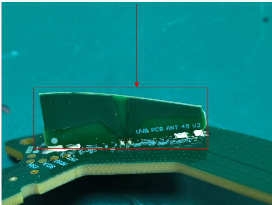
R-UWB ANT
