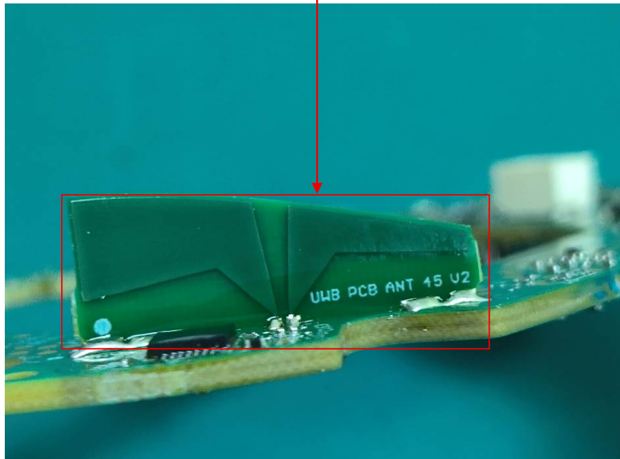
L-UWB ANT
