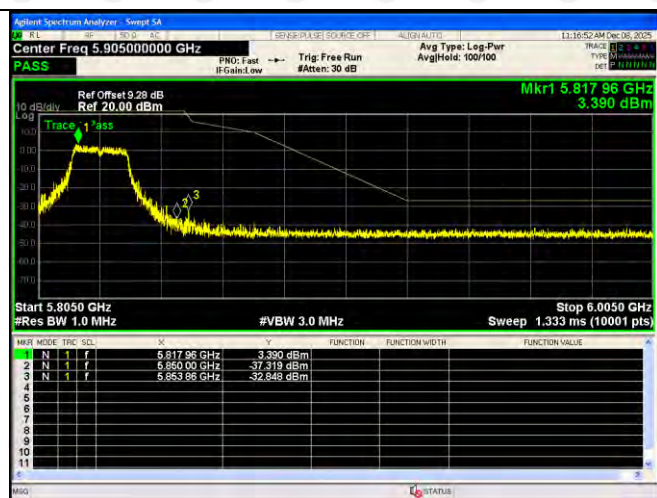
802.11(n40)-5795
