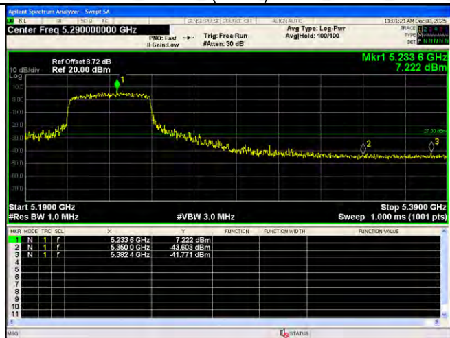
802.11ax(HE40)-5230
