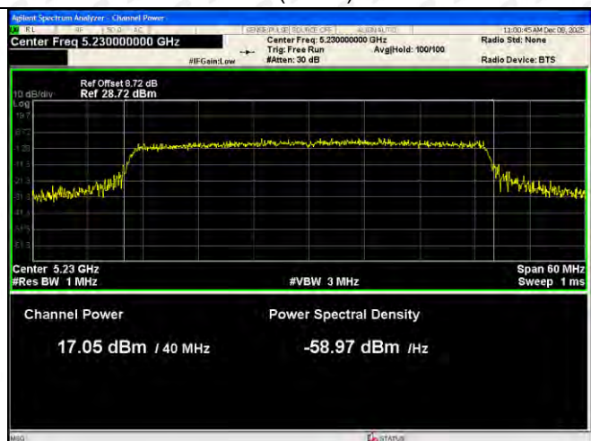
802.11ax(HE40)-5230
