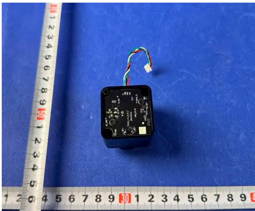
Figure 34. Lidar Motor
