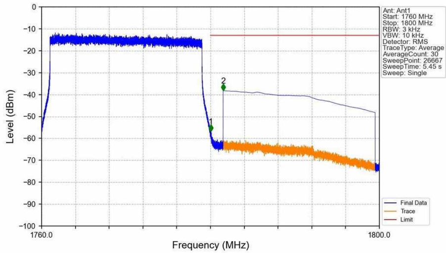
Band66_20MHz_16QAM_HCH_1770MHz_RB_1_99_NTNV
