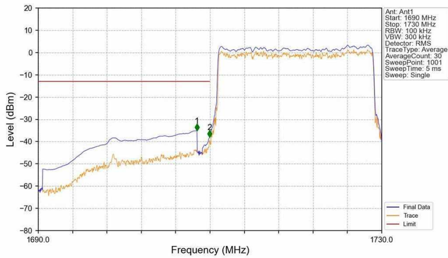
Band66_20MHz_QPSK_LCH_1720MHz_RB_100_0_NTNV
