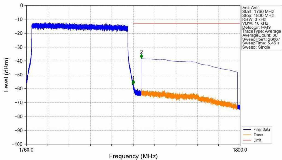
Band66_20MHz_QPSK_HCH_1770MHz_RB_1_99_NTNV
