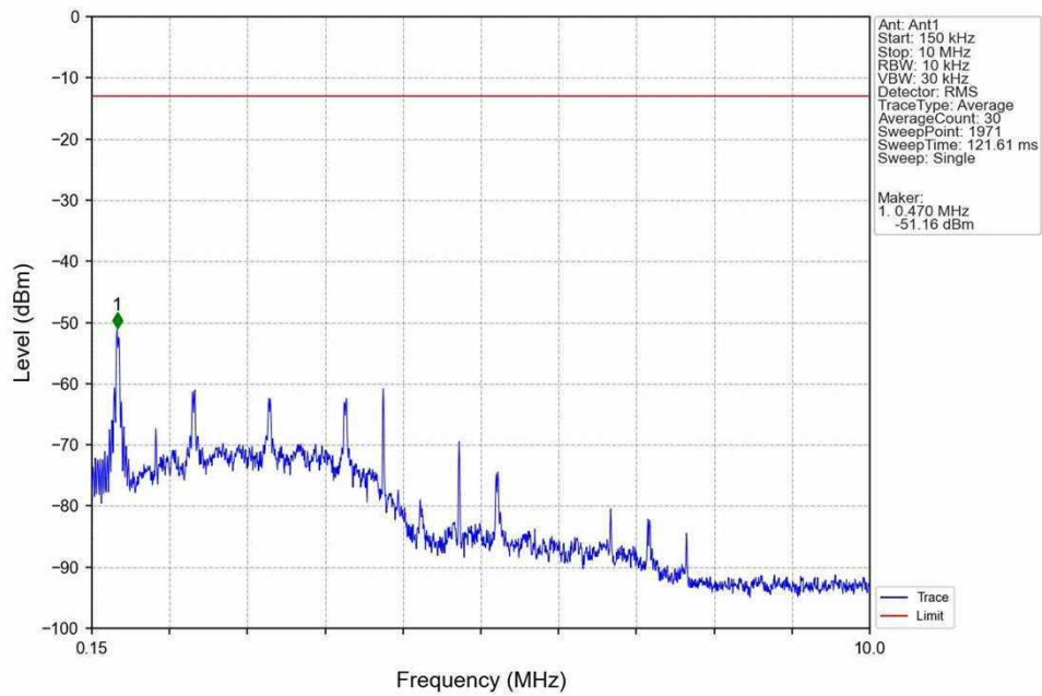
Band5_HSUPA_MCH_836.6MHz_Subtest 1_NTNV
