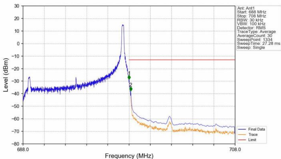
Band71_10MHz_QPSK_HCH_693MHz_RB_1_49_NTNV
