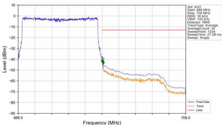
Band71_10MHz_QPSK_HCH_693MHz_RB_50_0_NTNV
