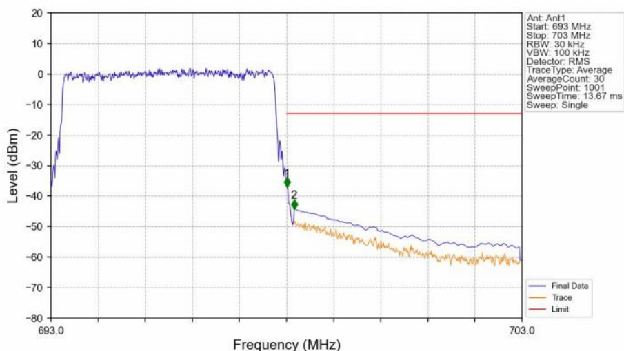
Band71_5MHz_QPSK_HCH_695.5MHz_RB_25_0_NTNV
