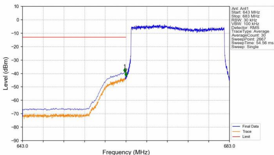
Band71_20MHz_16QAM_LCH_673MHz_RB_100_0_NTNV
