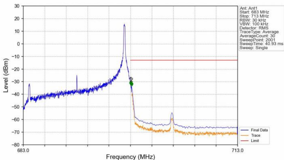
Band71_15MHz_QPSK_HCH_690.5MHz_RB_1_74_NTNV
