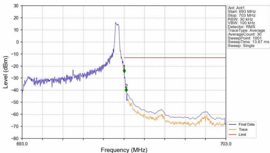
Band71_5MHz_QPSK_HCH_695.5MHz_RB_1_24_NTNV
