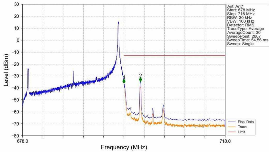
Band71_20MHz_QPSK_HCH_688MHz_RB_1_99_NTNV
