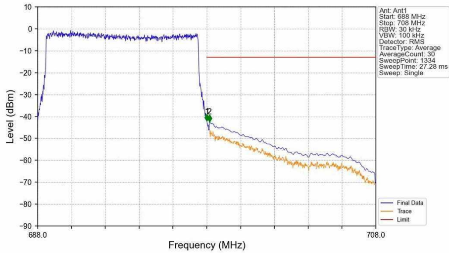
Band71_10MHz_QPSK_HCH_693MHz_RB_1_49_NTNV
