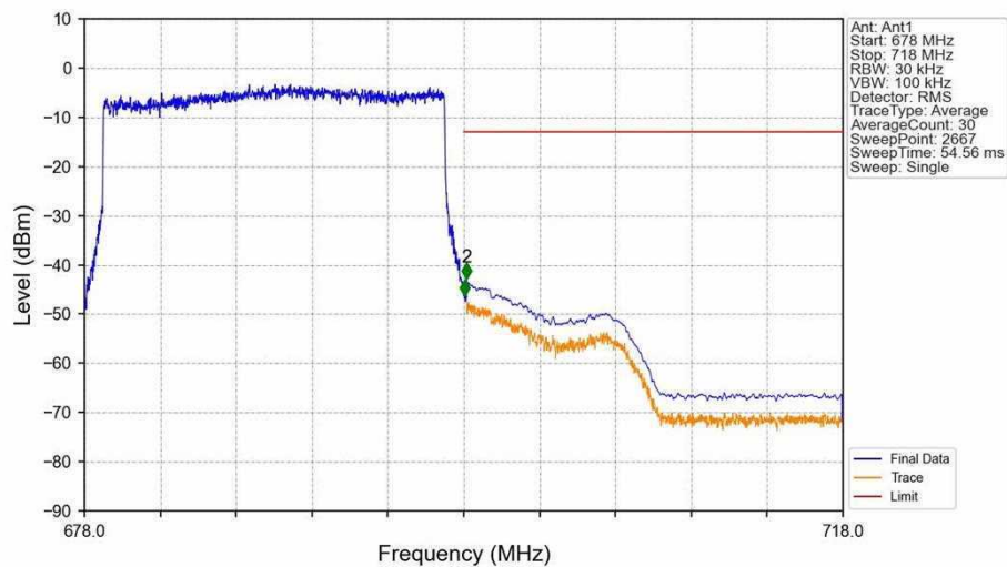
Band71_20MHz_QPSK_HCH_688MHz_RB_100_0_NTNV
