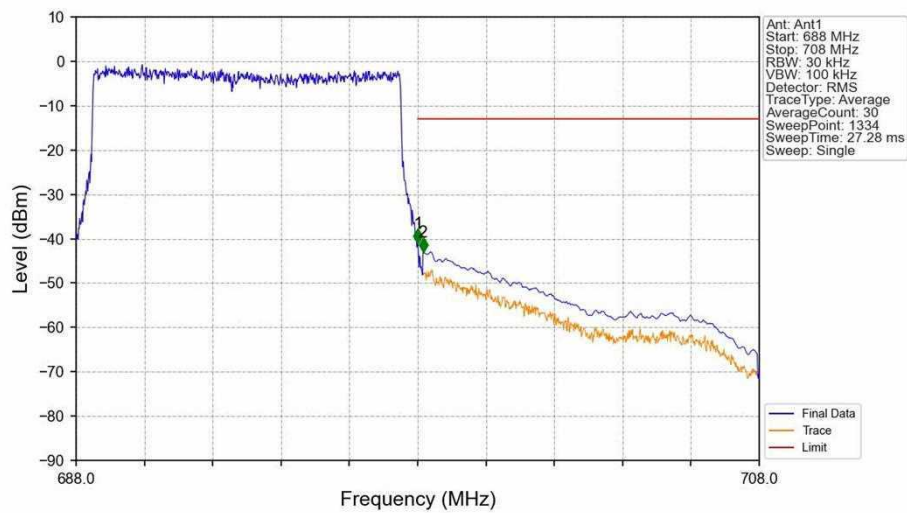
Band71_10MHz_QPSK_HCH_693MHz_RB_50_0_NTNV
