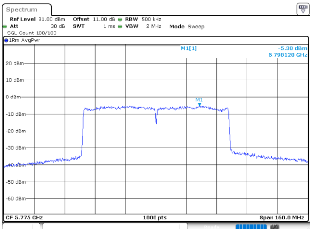
802.11ac80_5775MHz
