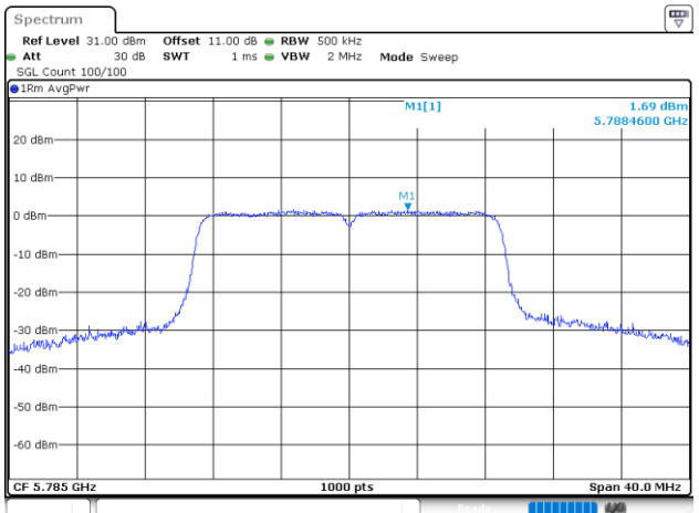
802.11ac20_5785MHz
